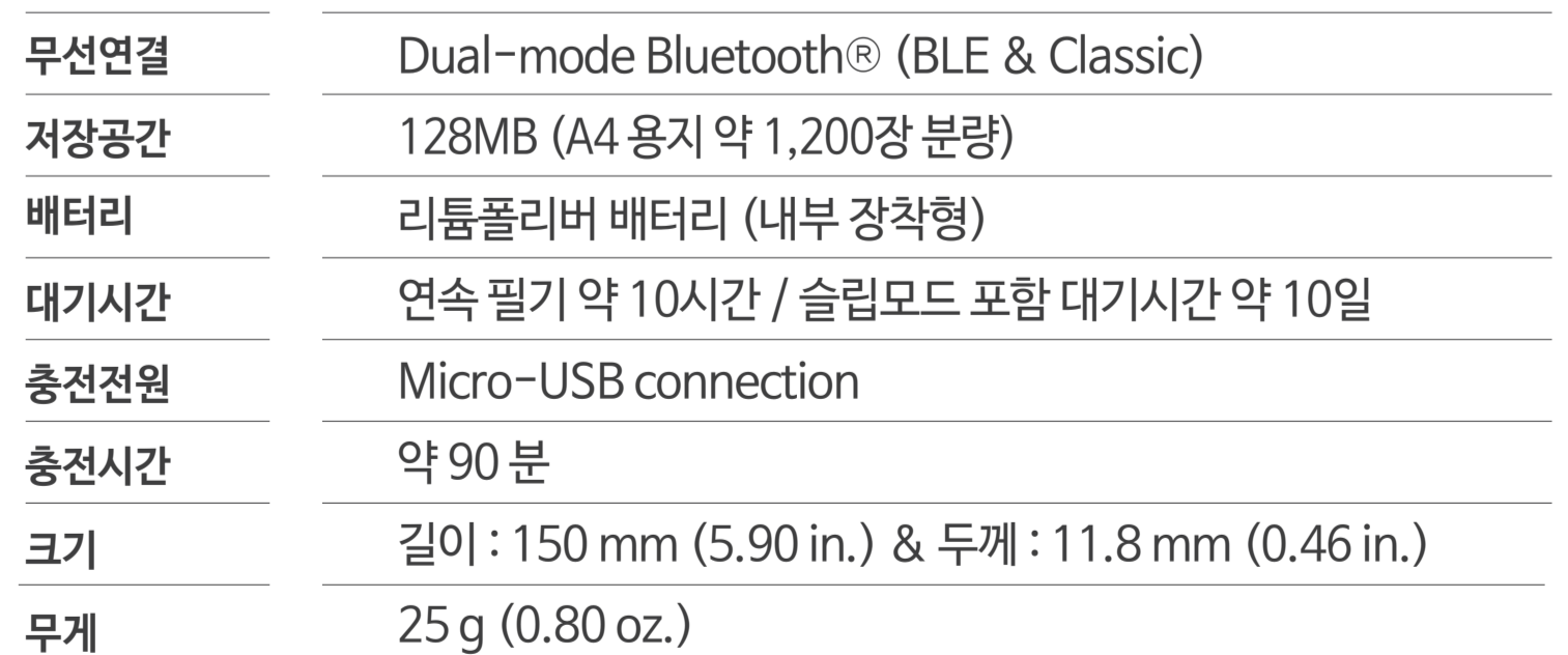
AP-701C Aegir
